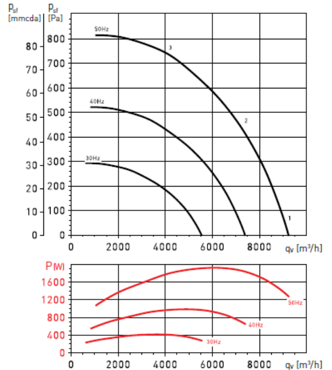
CHAT/4-560N 1,5kW
