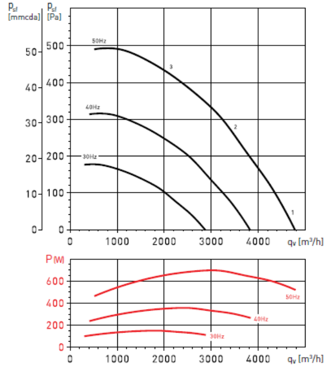
CHAT/4-450N 0,55kW
