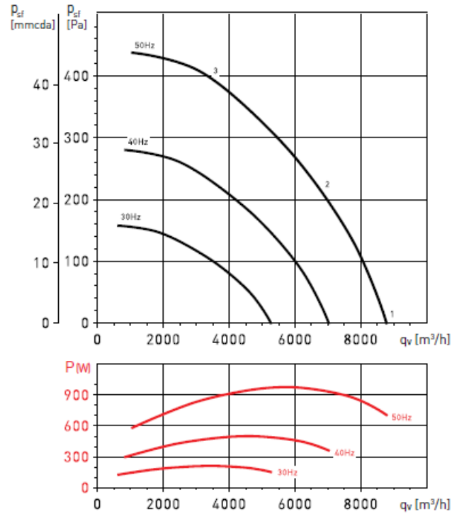
CHAT/6-630N 1,1kW
