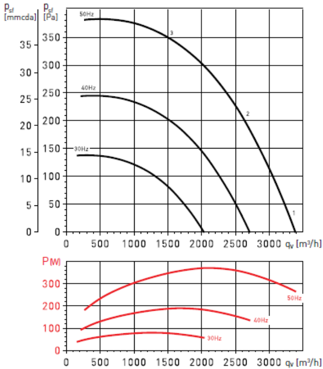
CHAT/4-400N 0,37kW
