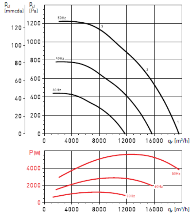
CHAT/4-710N 5,5kW
