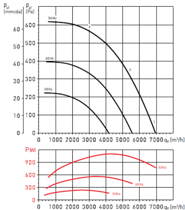
CHAT/4-500N 1,1kW
