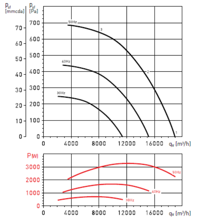
CHAT/6-800N 3kW
