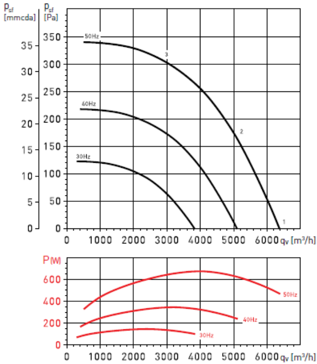
CHAT/6-560N 0,55kW
