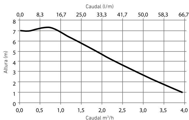
Curva del circulador incluido
