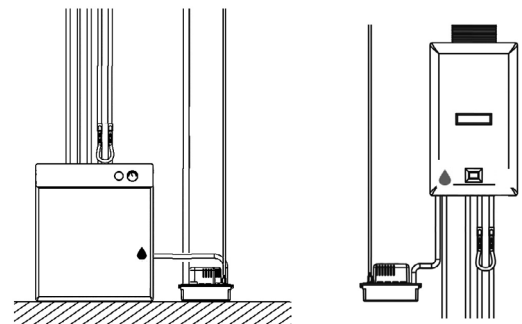
Conexiones hidráulicas
