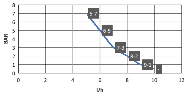
Presión (bar) - Caudal (l/h)
