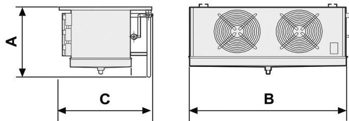
Evaporadores cúbicos
