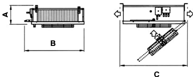
Doble flujo
