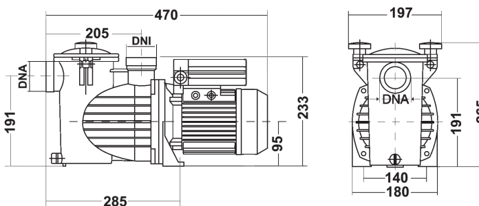
Dimensiones bomba
