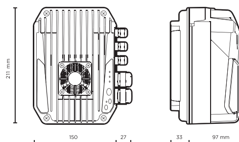
Dimensiones inversor
