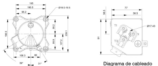
Diagrama de cableado
