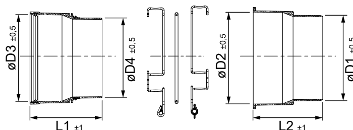
Manguito hembra Ø160/Ø200
