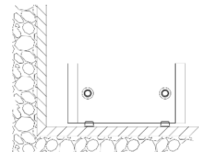
Instalación horizontal sobre soportes
