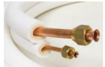
Detalle del abocardado y tuerca
