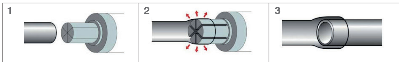
Cabezas para tenaza expandidora
