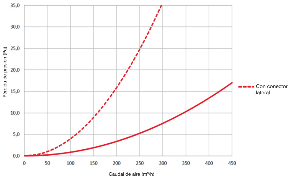
Pérdida de carga - Conector lateral
