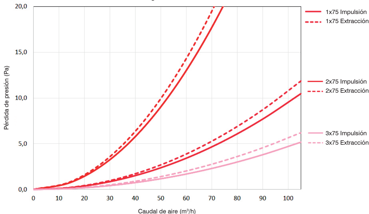
Pérdida de carga - Plenum 3x75 HEATPEX ARIA
