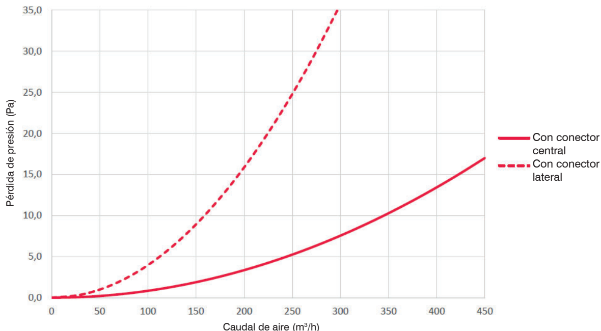
Pérdida de carga - Caja de distribución 10x75
