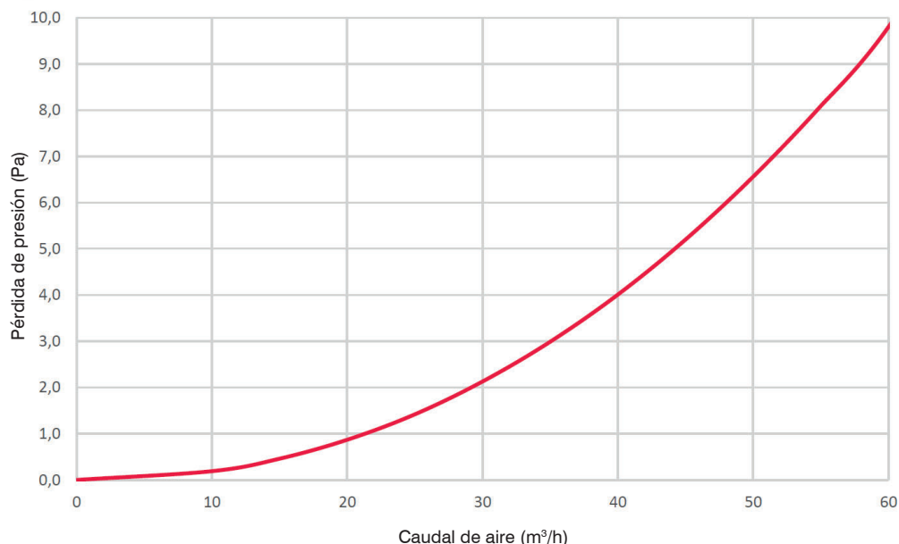
Pérdida de carga - Conducto 75 HEATPEX ARIA
