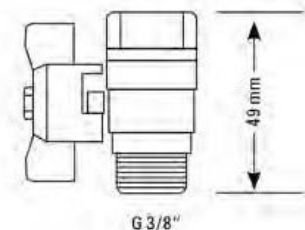
Válvula de bola de cierre G 3/8" acero inoxidable
