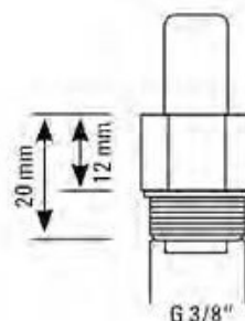
Con junta Ryton Junta Vitón 13x2 Junta Vitón inserción 7x2
