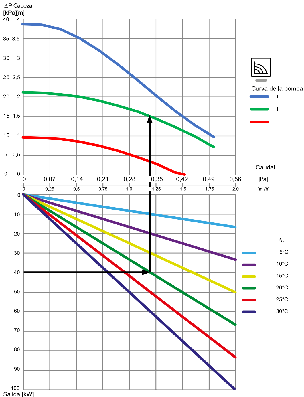
LTC341 – presión disponible de la bomba, velocidad constante
