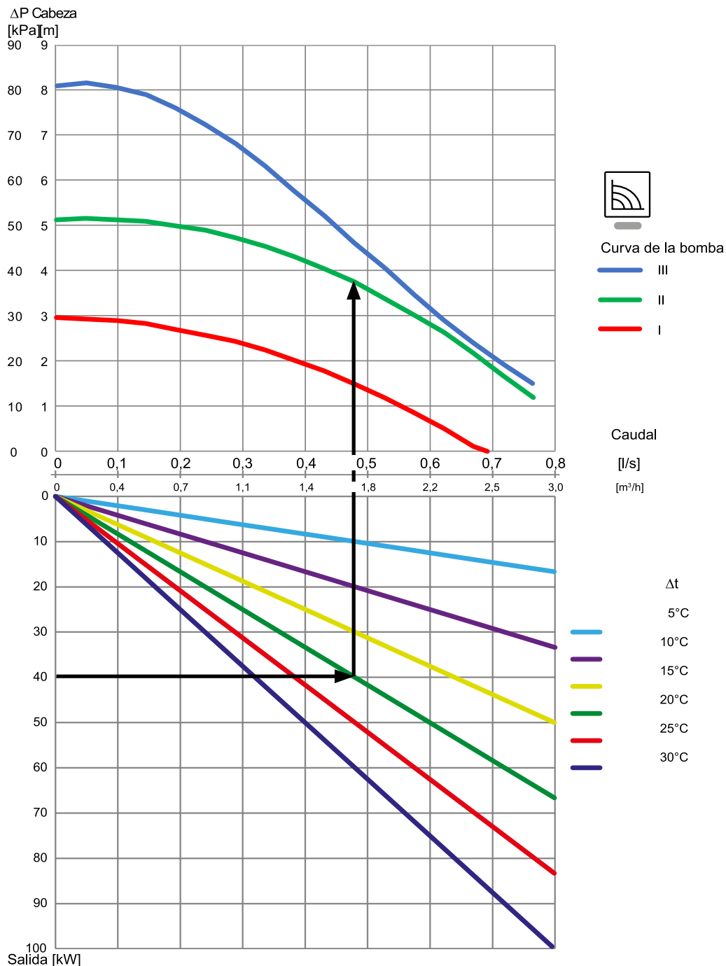
LTC381 – presión disponible de la bomba, velocidad constante
