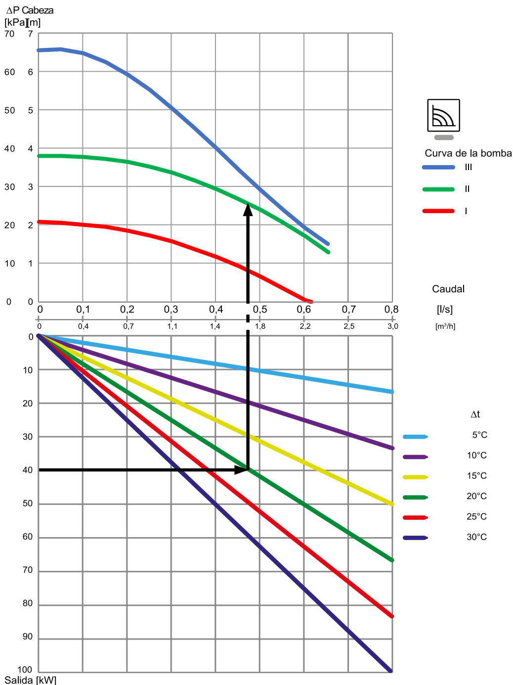
LTC361 – presión disponible de la bomba, velocidad constante
