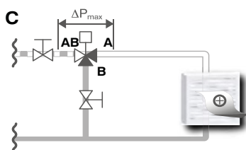
Instalación sin bomba de circulación local
