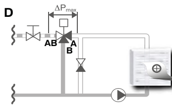
Instalación con bomba de circulación local
