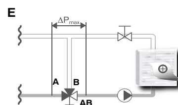
Instalación con bomba de circulación local
