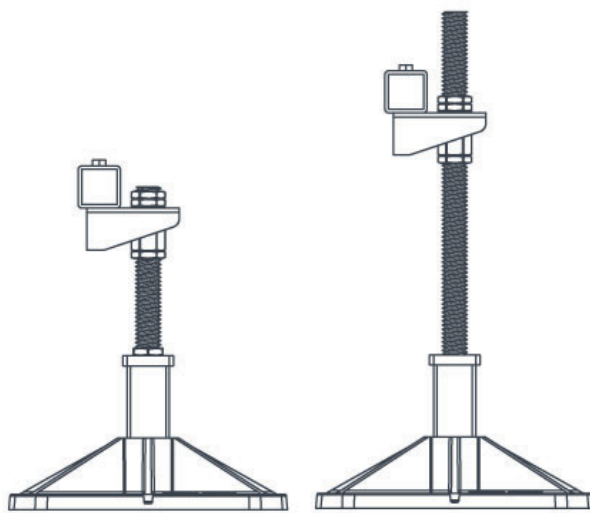
Base y Standard Ajuste de altura: 335 - 440mm
