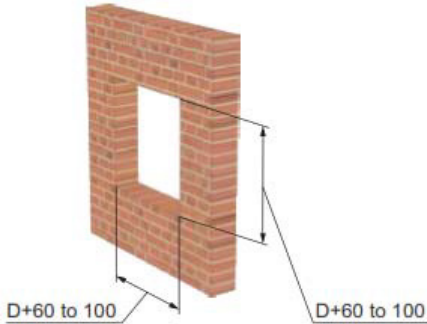
1. Abertura en obra soporte
