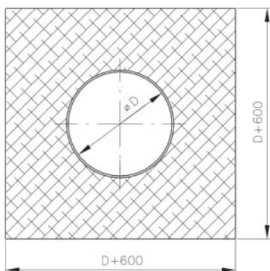
Fig. 3 Abertura en obra soporte Placas de lana mineral con revestimiento resistente al fuego
