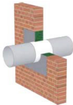
5. Aplicar el sellador resistente al fuego a cada lado
