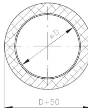
Fig. 2 Abertura en obra soporte
