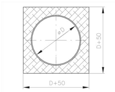
Fig. 1 Abertura en obra soporte
