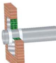
3. Rellenar el hueco y cubrir el conducto con recubrimiento cortafuegos
