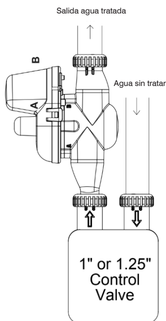
Instalación directa en válvula Clack
