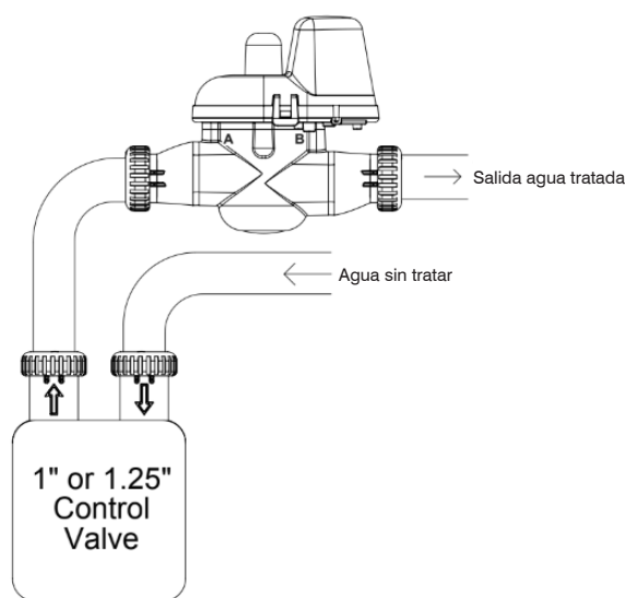
Instalación separada de válvula clack con los correspondientes racores
