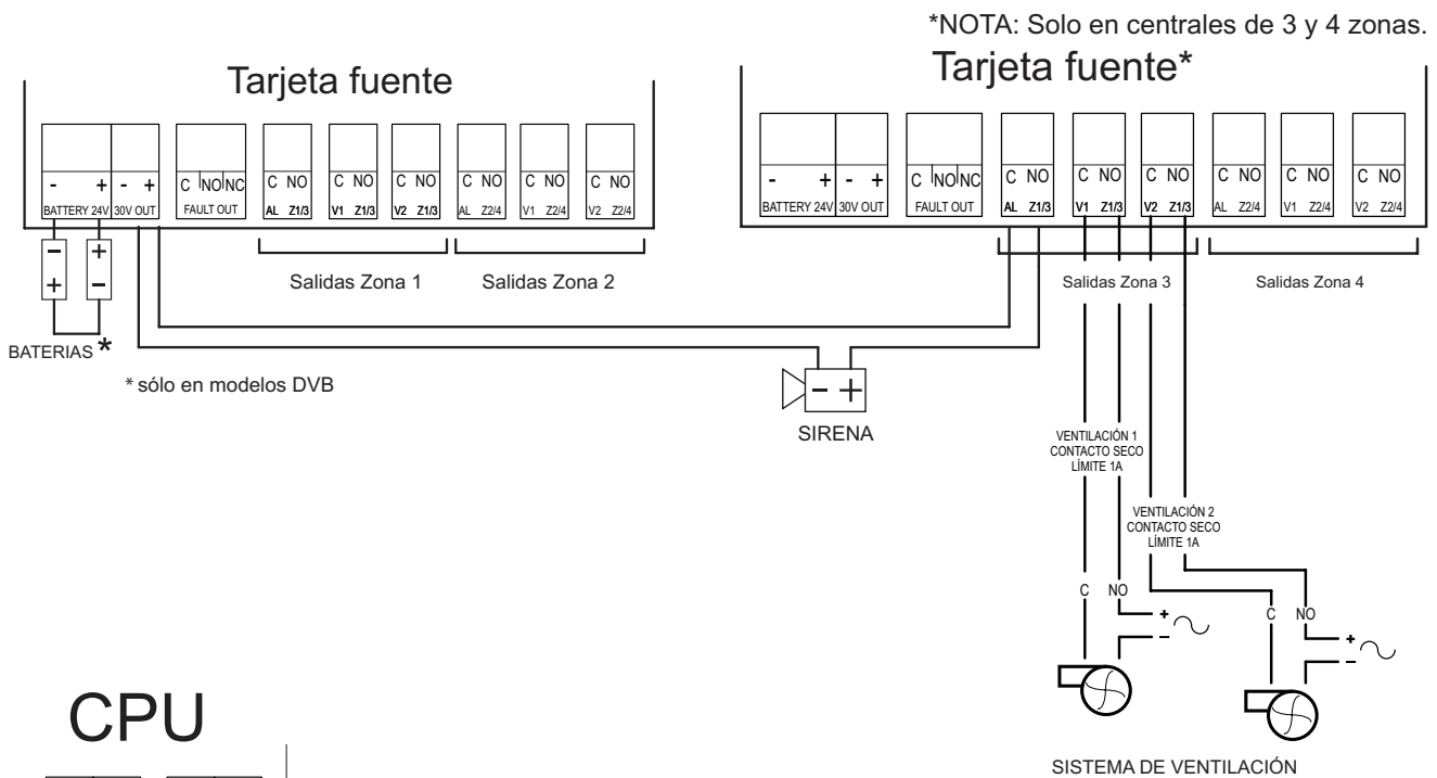
Esquema de funcionamiento para centrales DVB
