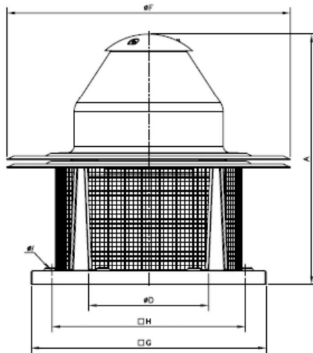
Modelo CHT
