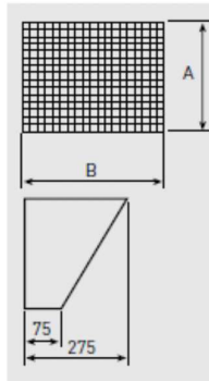
Dimensiones (mm)
