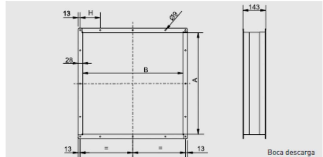
Boca descarga
