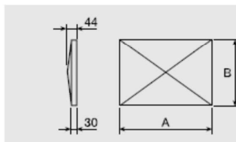
CHTI Tapa intemperie para modelos de descarga horizontal para protección de instalaciones en el exterior.
