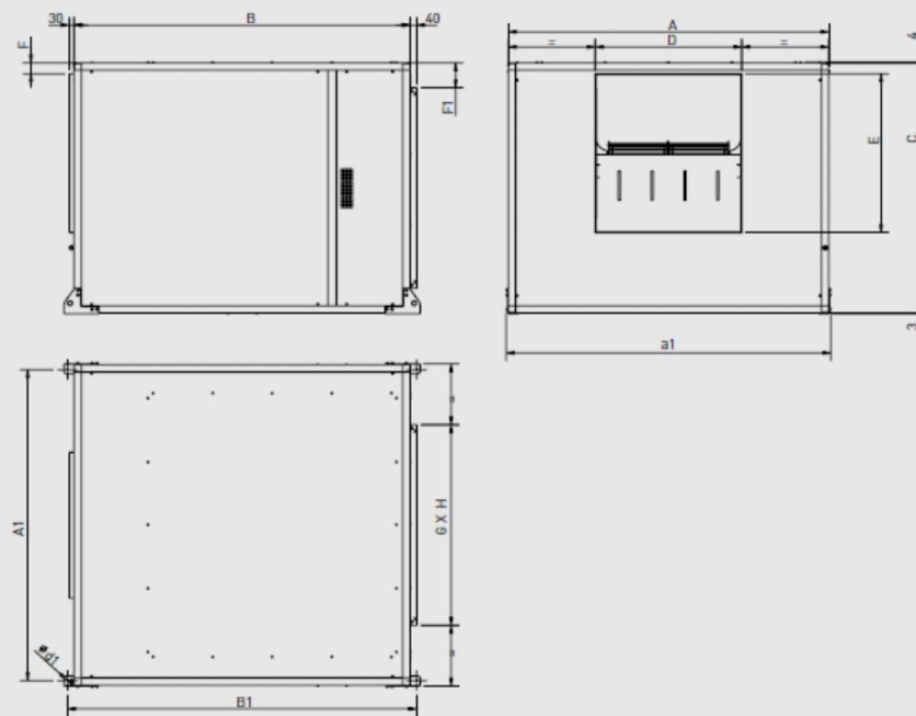
CVHT 20-22-25-30 Horizontal
