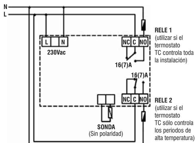
Esquema conexionado termostato TC
